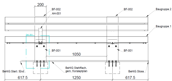
Draufsicht Mst. (1:16)
