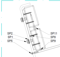
Det. 003 (1:5)
