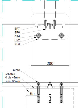
Det. 001 (1:5)
