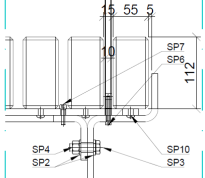
Det. 003 (1:5)
