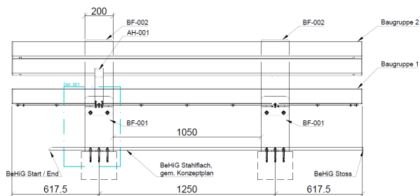
Draufsicht Mst. (1:16)
