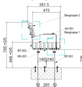
Det. 001 (1:5)
