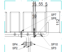
Det. 003 (1:5)
