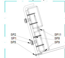
Det. 003 (1:5)
