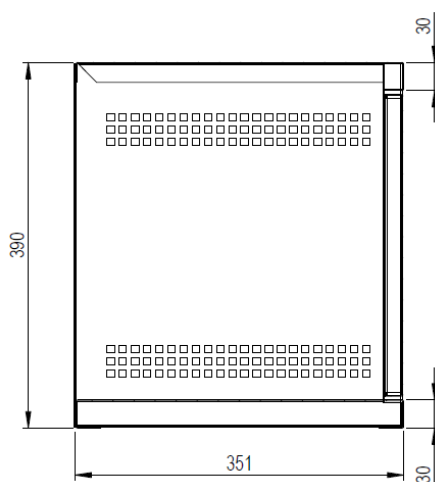
Seitenansicht
